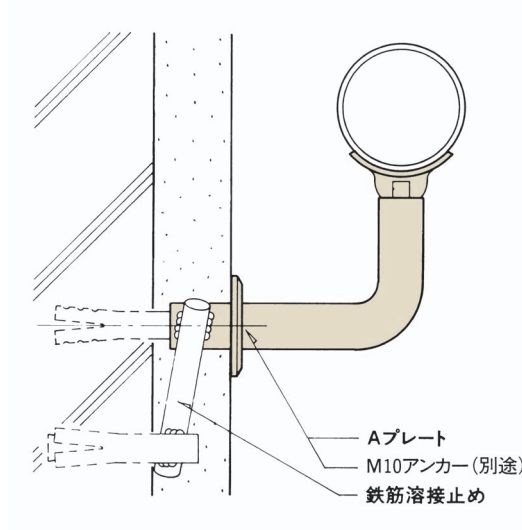
Aプレートコンクリート下地取付詳細図
