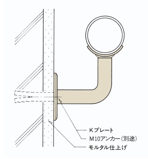
Kプレートモルタル下地取付詳細図
