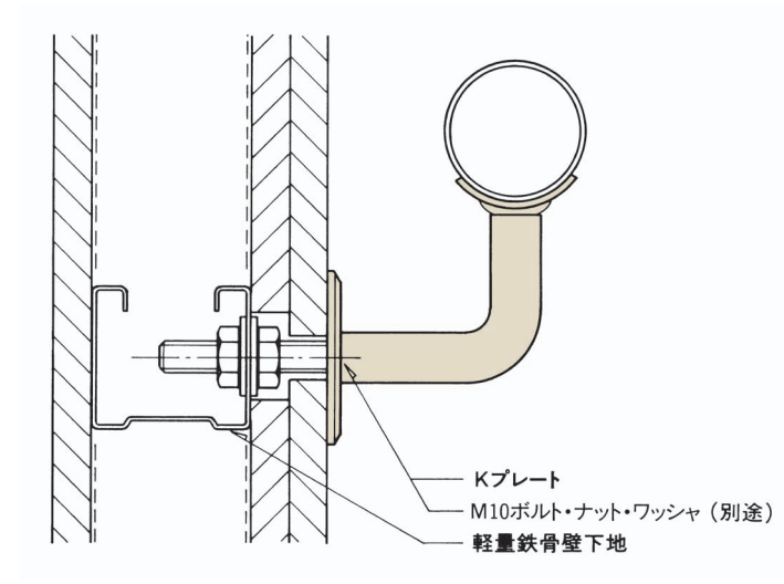
Kプレート軽量鉄骨壁下地取付詳細図
