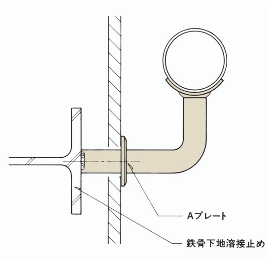
Aプレート鉄骨下地取付詳細図
