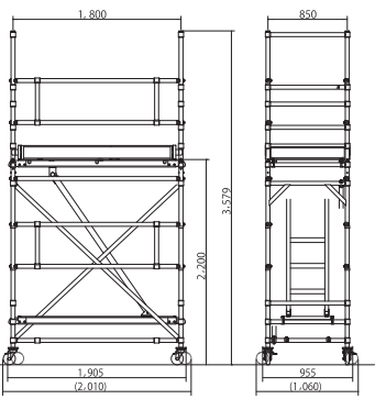
作業床高さ2200mm状態
