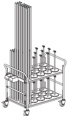
NT-WGK-1 (ベース&バータイプ) 専用ワゴン(詳細は、P77参照)
