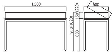
展示ケース・STF-15060 (15060-2)
