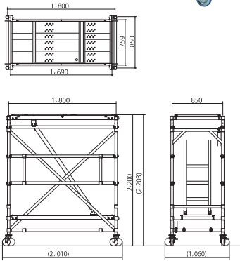
2200mm収納状態
